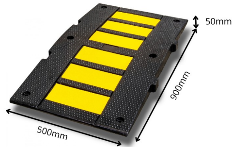
KSC900 Body Module
